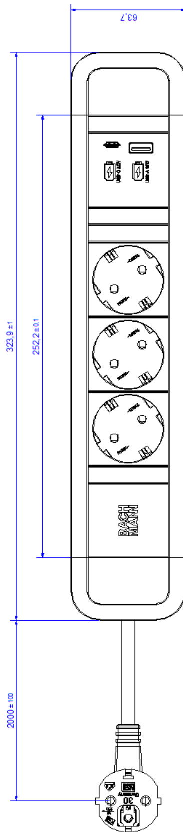
H05VV-F 3G 1,5mm 2 schwarz / black mit Winkelstecker CEE 7/7 / with angled plug CEE 7/7
