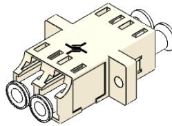
J08071A0010 Gehäuse beige / Housing beige
