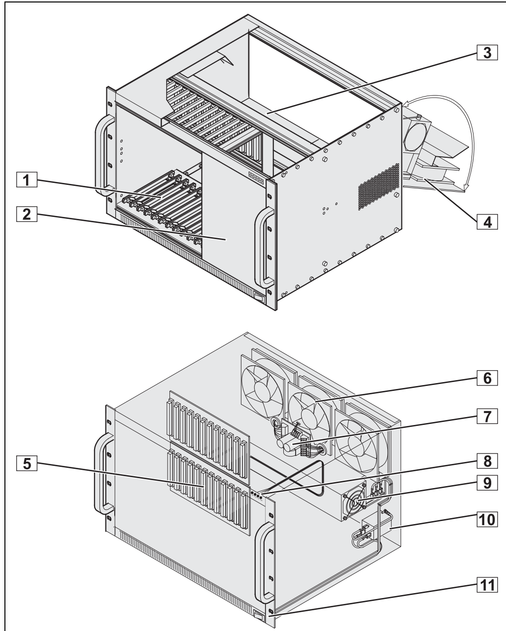
Figure 1: Einschubsystem Übersicht
