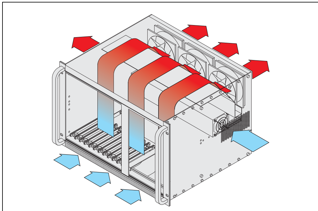
Figure 4: Entwärmung
